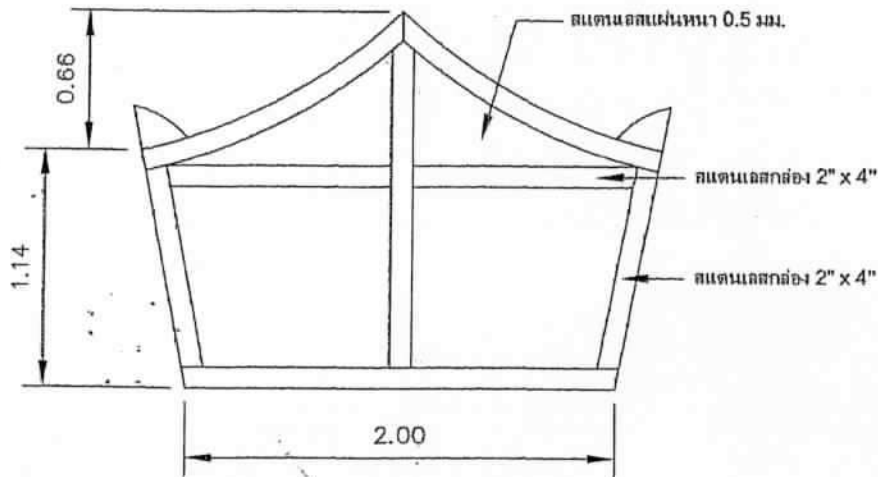
แบบขยายโครงสร้างป้าย SCALE 1:25
