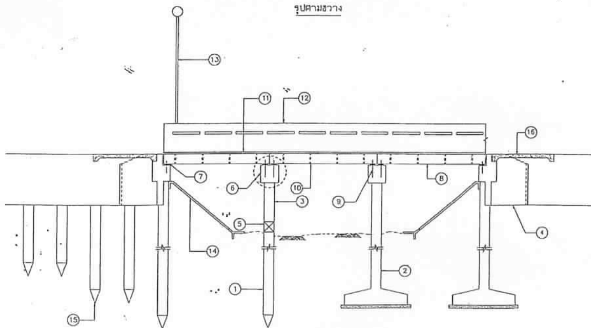
รูปตามยาว
