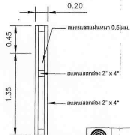
รูปด้านข้างป้าย SCALE 1:25
