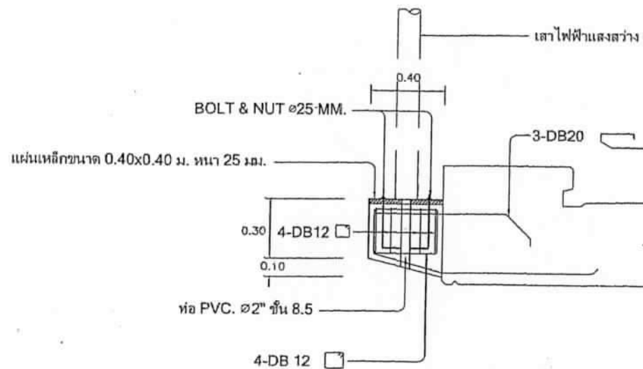
แบบขยายแท่นติดตั้งเสาไฟฟ้า SCALE 1:20
