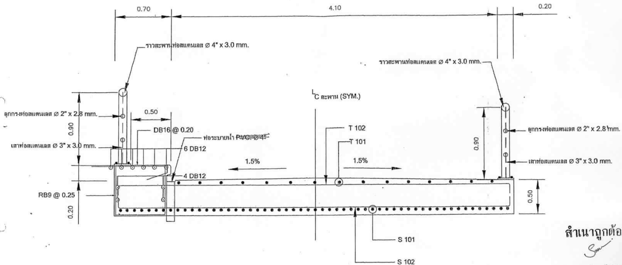
แบบขยายพื้นสะพาน SCALE 1:20
