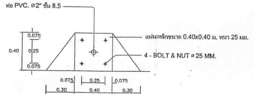
แปลนแท่นติดตั้งเสาไฟฟ้า SCALE 1:20
