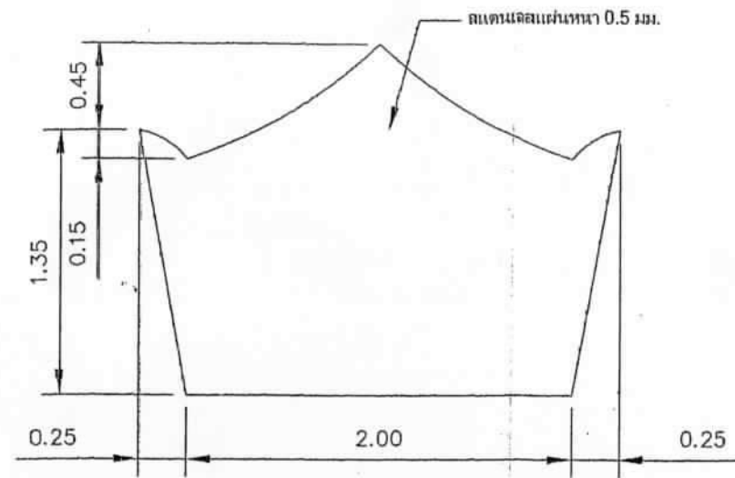
รูปด้านหลังป้าย SCALE 1:25
