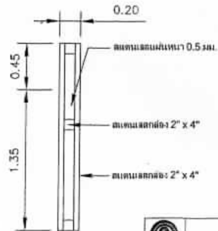
รูปด้านข้างซ้าย SCALE 1:25
