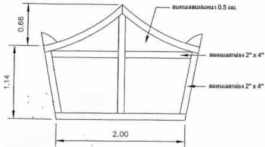
แบบขยายโครงสร้างบ้าน SCALE 1:25
