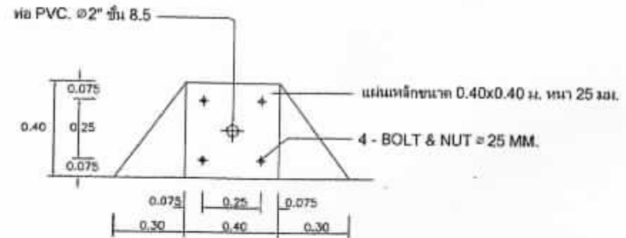
แปลนแท่นติดตั้งเสาไฟฟ้า SCALE 1:20
