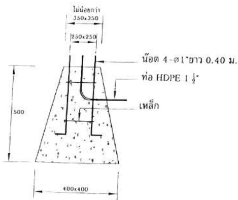
แบบขยายต่อม่อ
