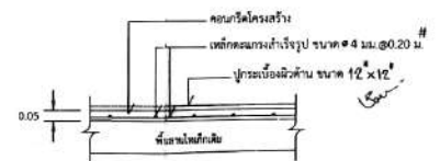
แบบขยายพื้น ค.ส.ล.ลานไถ่
